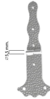
19101 30,5x11,5 cm Ø 44 kg. - 4 mm.
