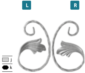
19070 9,5x15 cm 0,22 kg — 12x6 mm.
