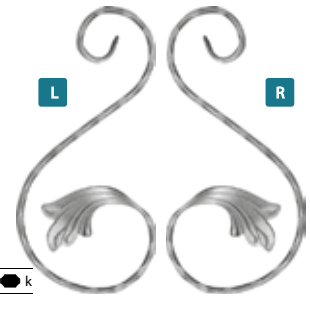
19236 13x25,5 cm 0,33 kg — 12x6 mm.
