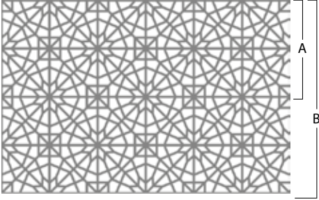
KM-03174 A 120x40 cm 5,23 kg / — 3 mm.
